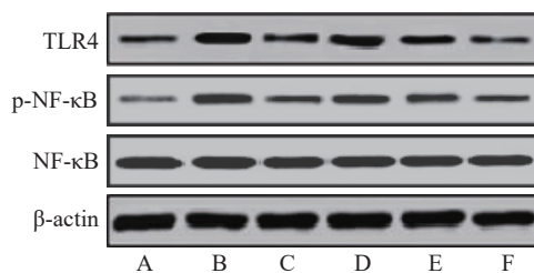
图3 各组大鼠缺血侧大脑皮层组织 TLR4、NF- \kappa B、p-NF- \kappa B 蛋白表达的比较
